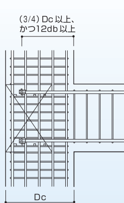
ト形柱梁接合部
