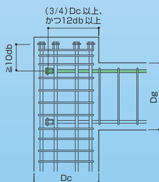
柱定着スタブ付き
