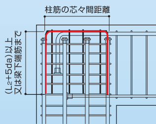
朝日式かんざし筋
