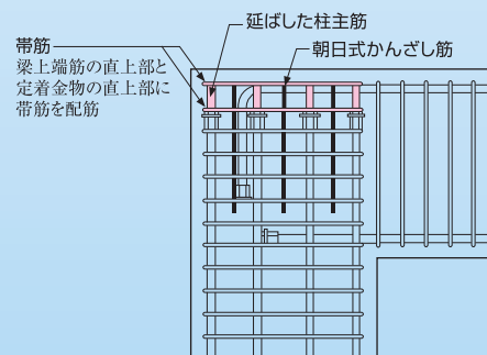
頭冠工法
