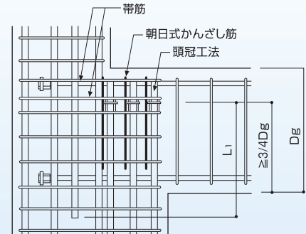
柱絞り部
