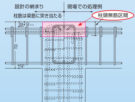
RC配筋指針 備考図9.8
