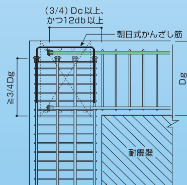
● 耐震壁付き
